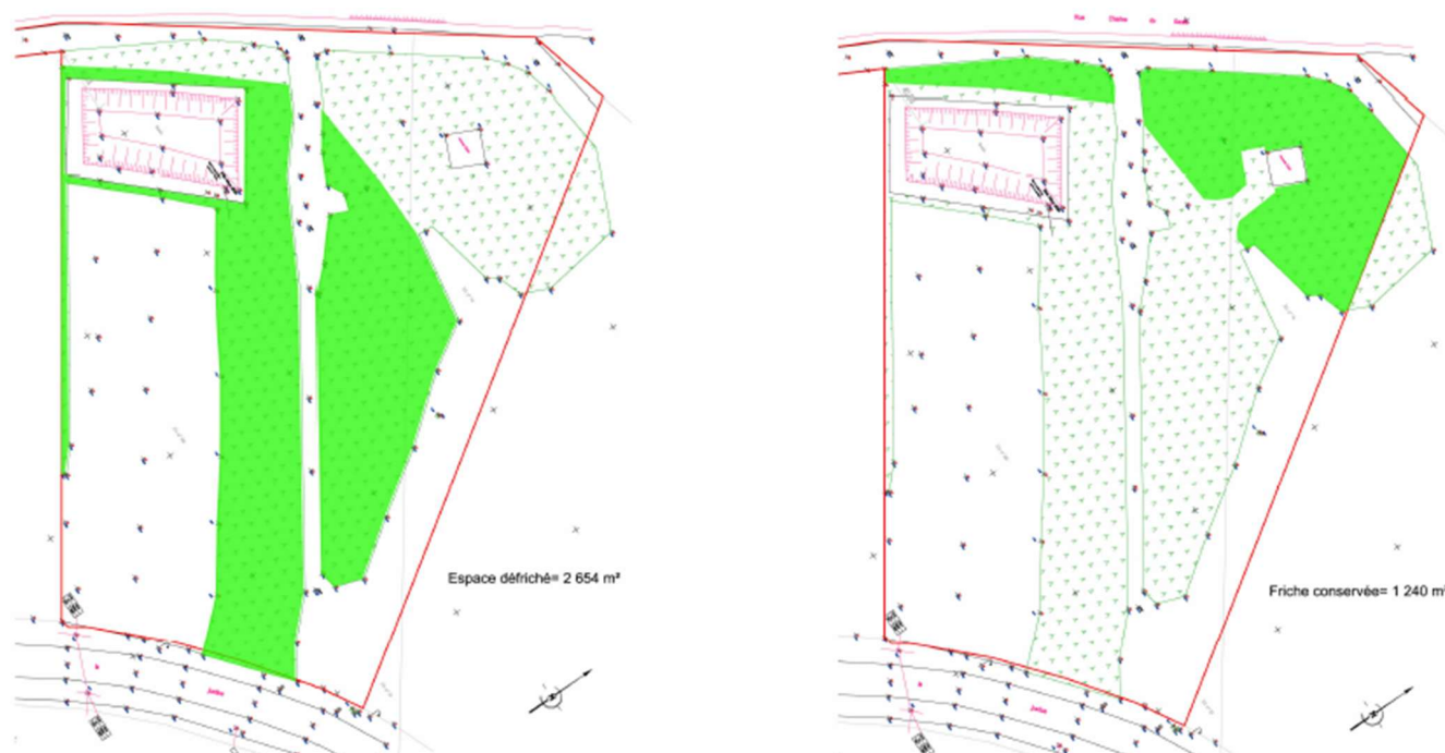
Figure 9 : Plan de défrichement du projet initial
