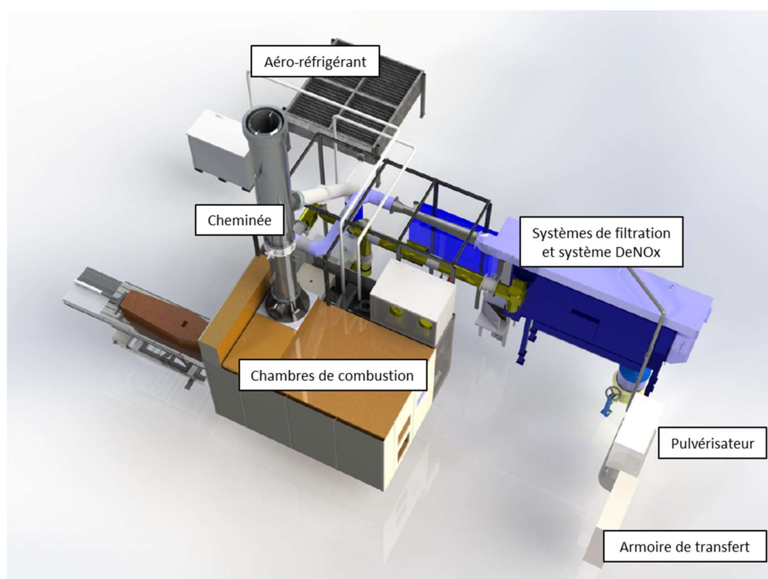
Figure 18 : Vue 3D du système de crémation
