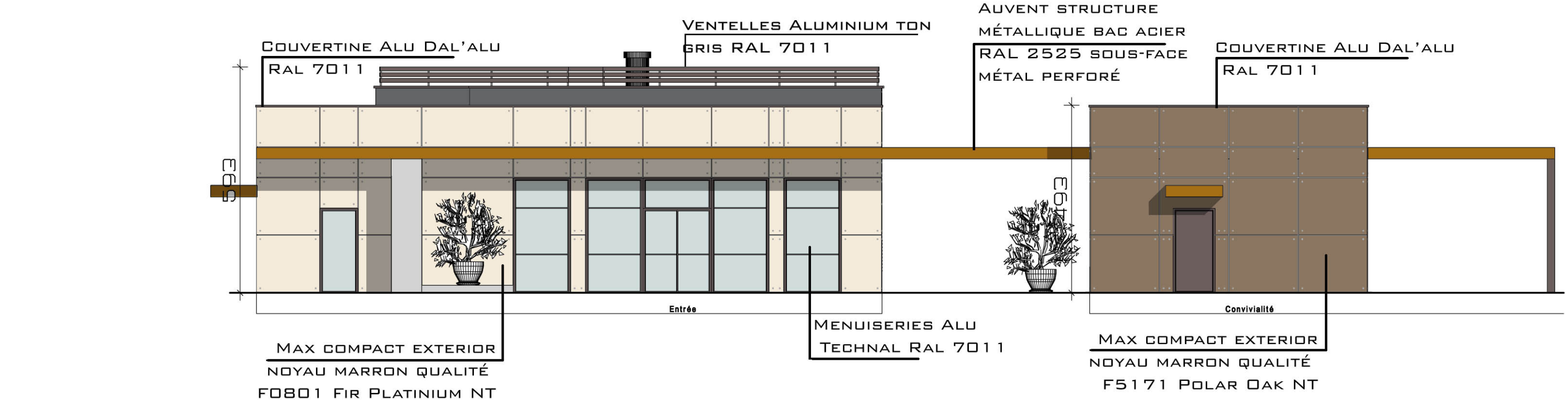
FAÇADE ENTRÉE (SUD)
