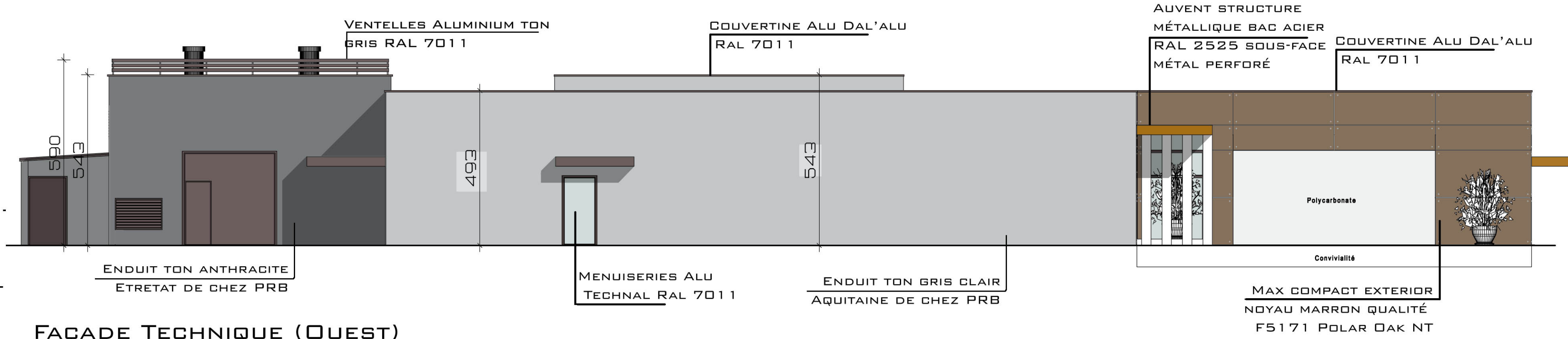
FAÇADE TECHNIQUE (OUEST)
